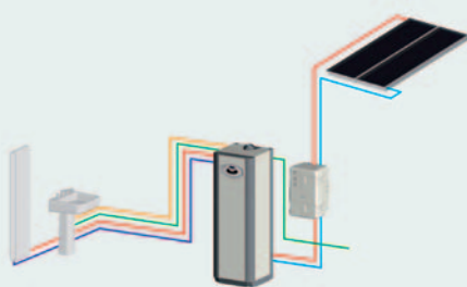
Příklad instalace
